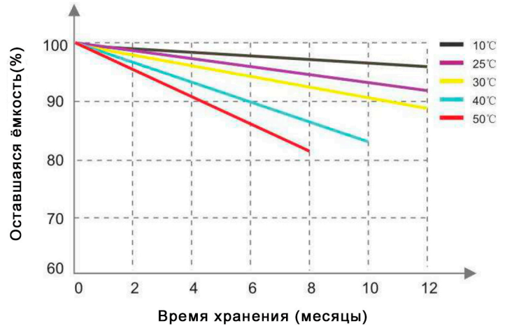
Кривая саморазряда при разной температуре
