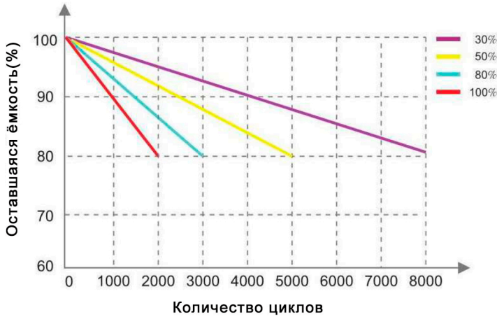
Кривая цикла разряда при разной DOD (0.5C)
